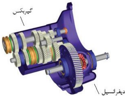
مجموعه گیربکس و دیفرانسیل
